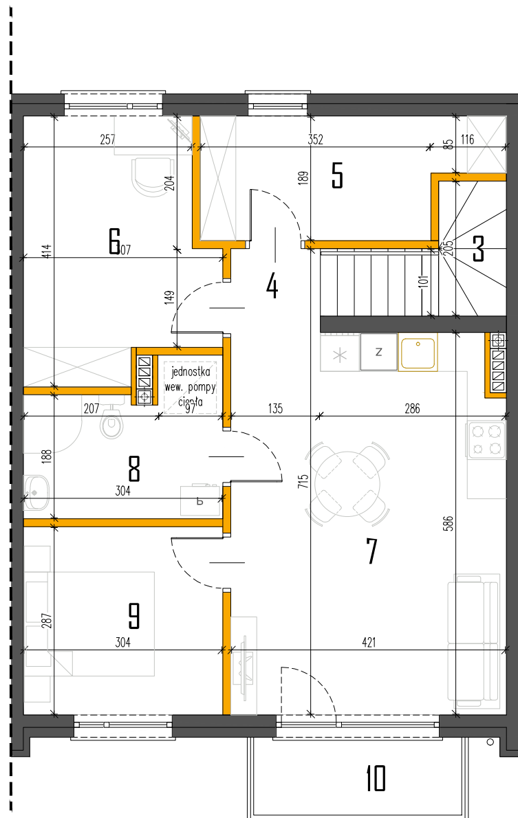
RZUT PIĘTRA
