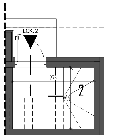
RZUT PARTERU
