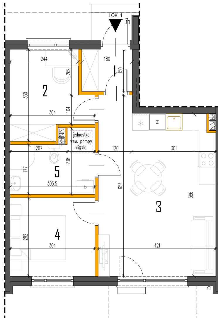
RZUT PARTERU
