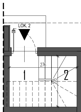
RZUT PARTERU
