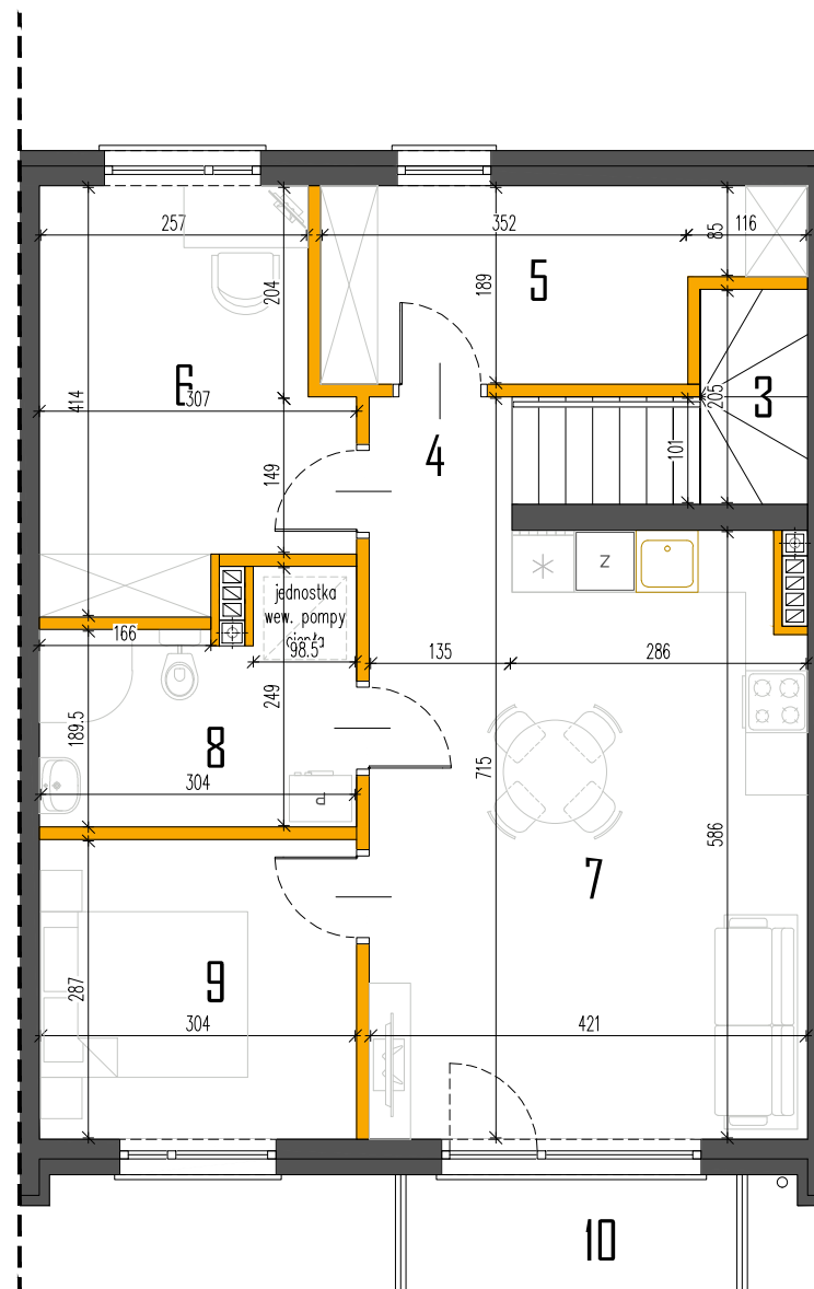
RZUT PIĘTRA
