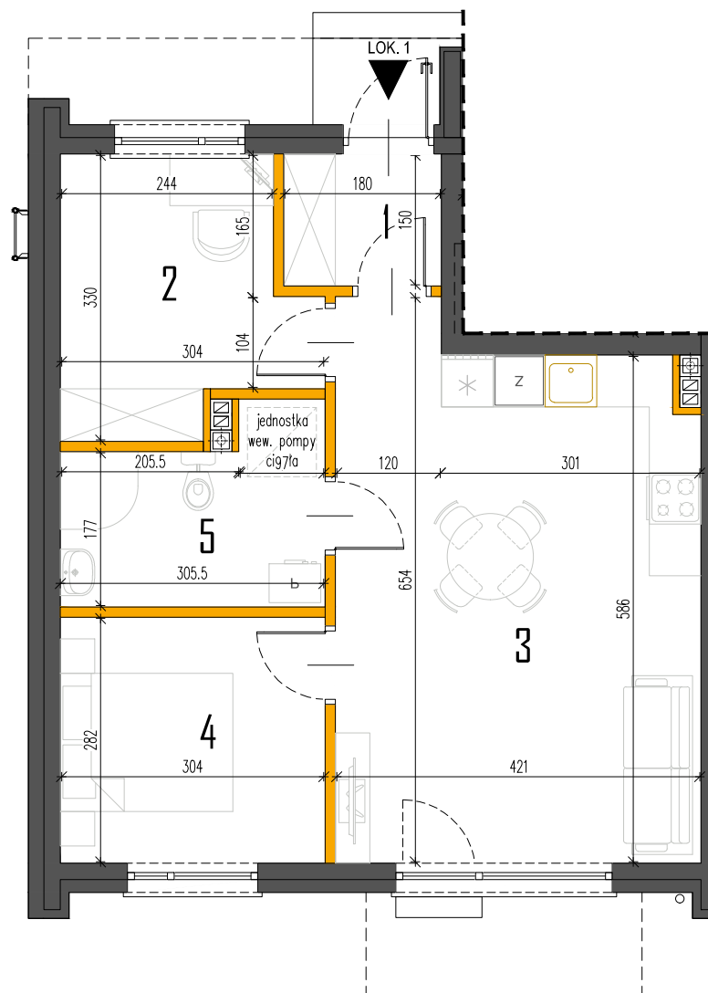
RZUT PARTERU
